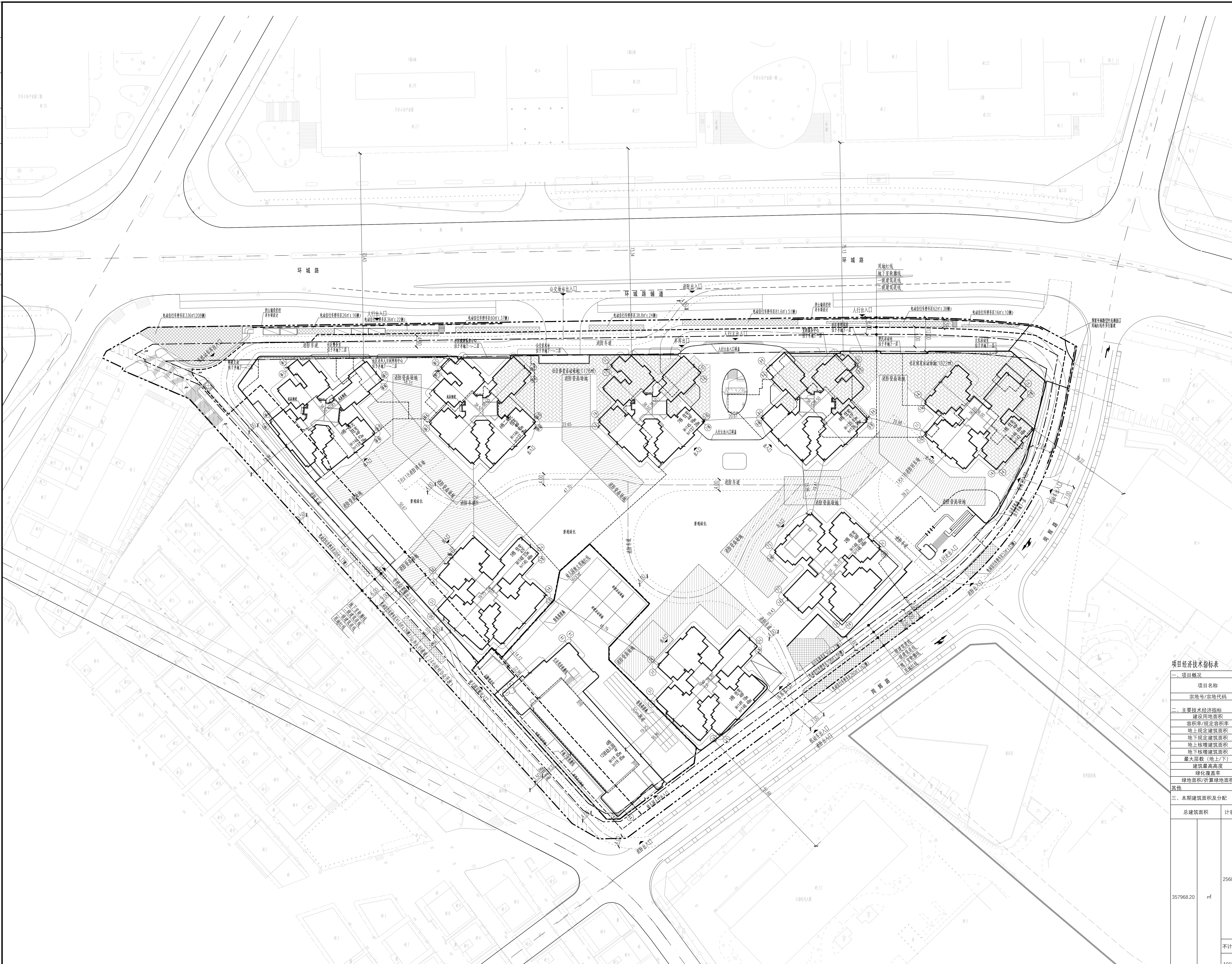
总平面图 1:500
