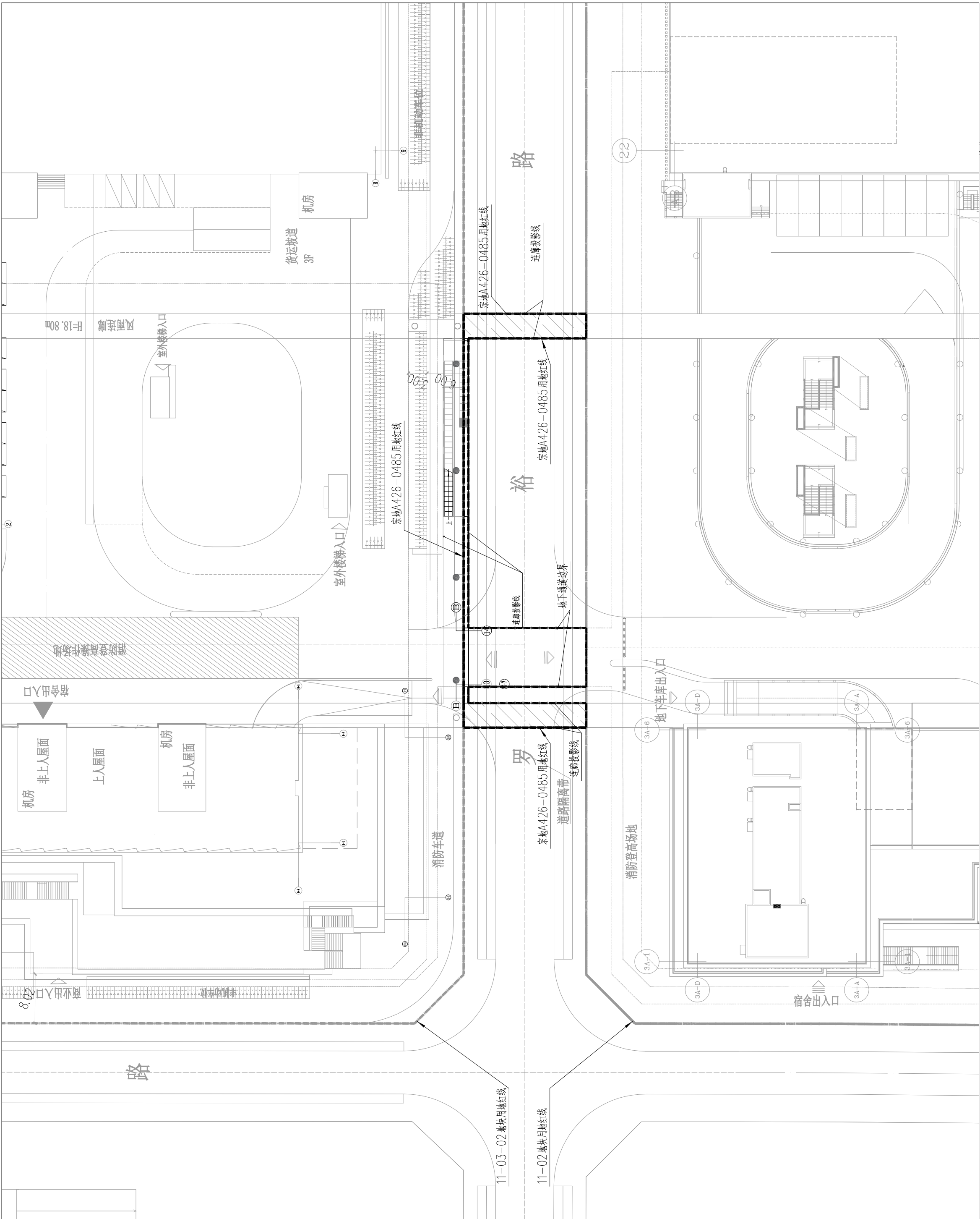
总平面图 1:500
