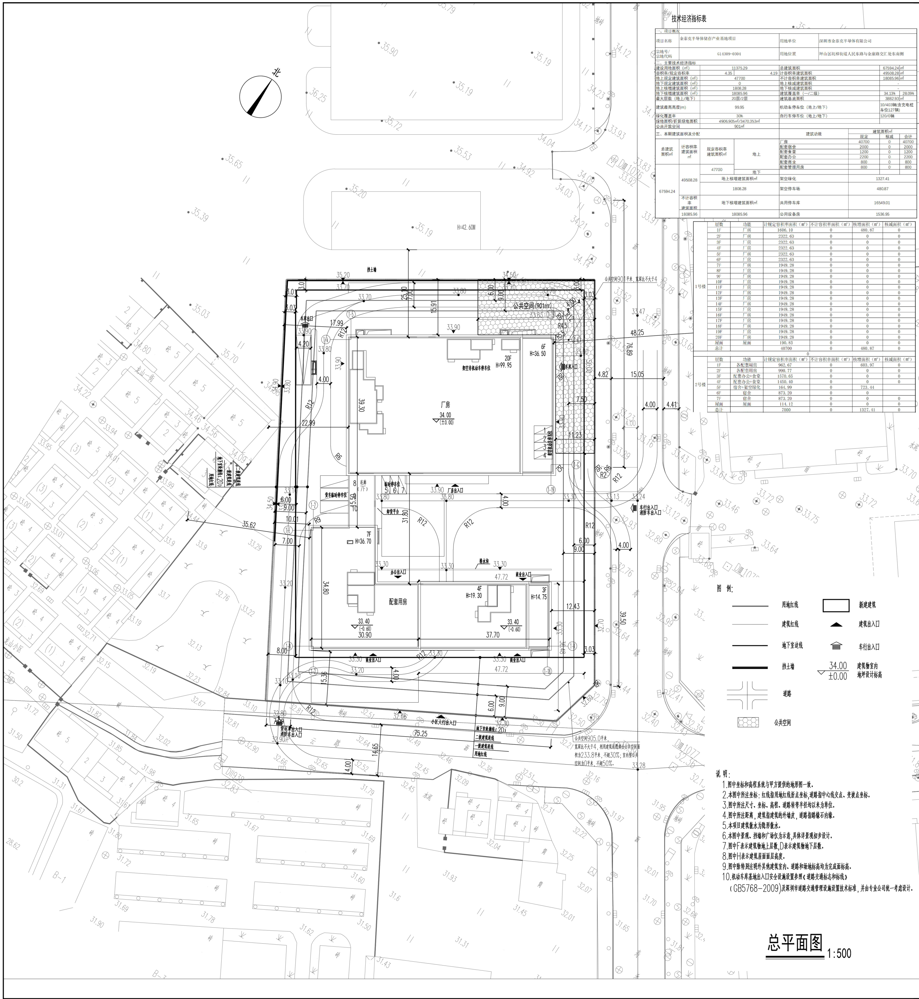
总平面图 (修改前)
