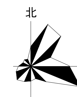
屋顶总平面图 1:500
