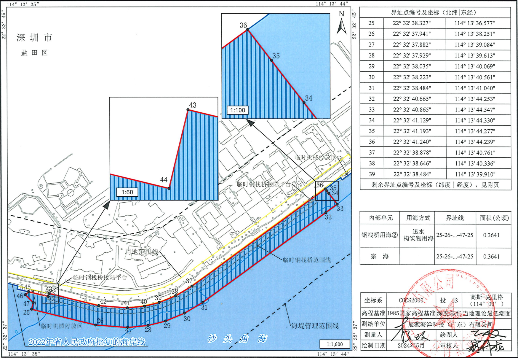
深圳市盐田区中英街海堤达标加固工程临时钢栈桥项目（钢栈桥用海②）宗海界址图
