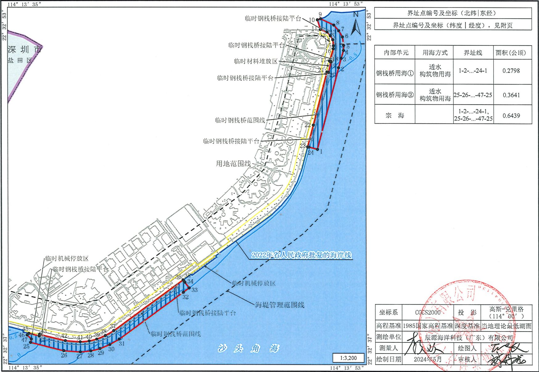
深圳市盐田区中英街海堤达标加固工程临时钢栈桥项目宗海界址总图
