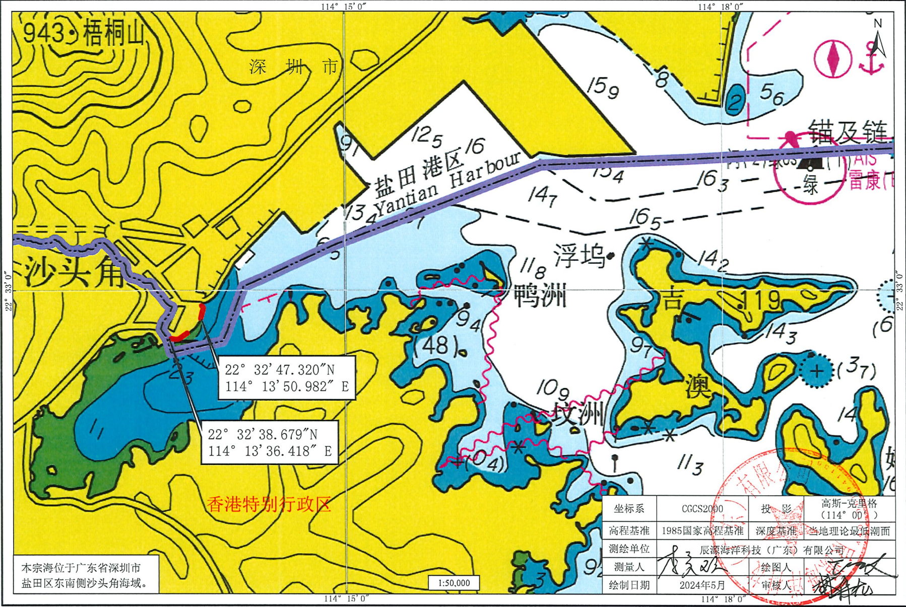
深圳市盐田区中英街海堤达标加固工程临时钢栈桥项目宗海位置图
