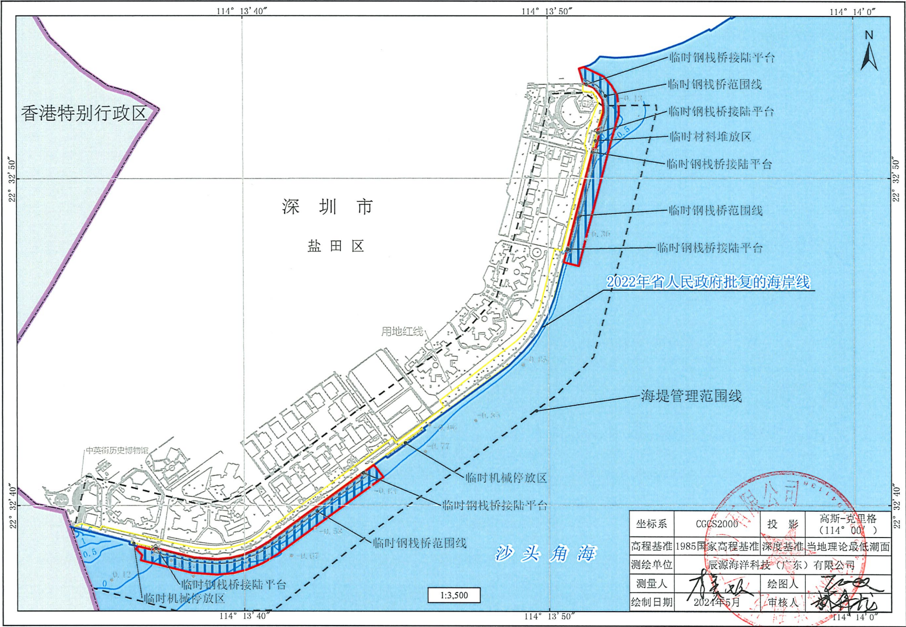
深圳市盐田区中英街海堤达标加固工程临时钢栈桥项目宗海平面布置图
