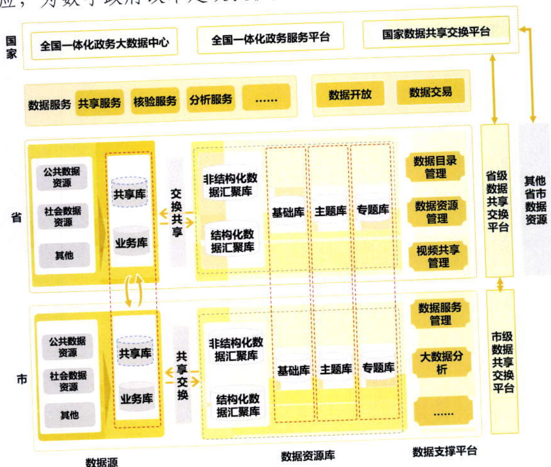
图 4 数字政府数据架构图
