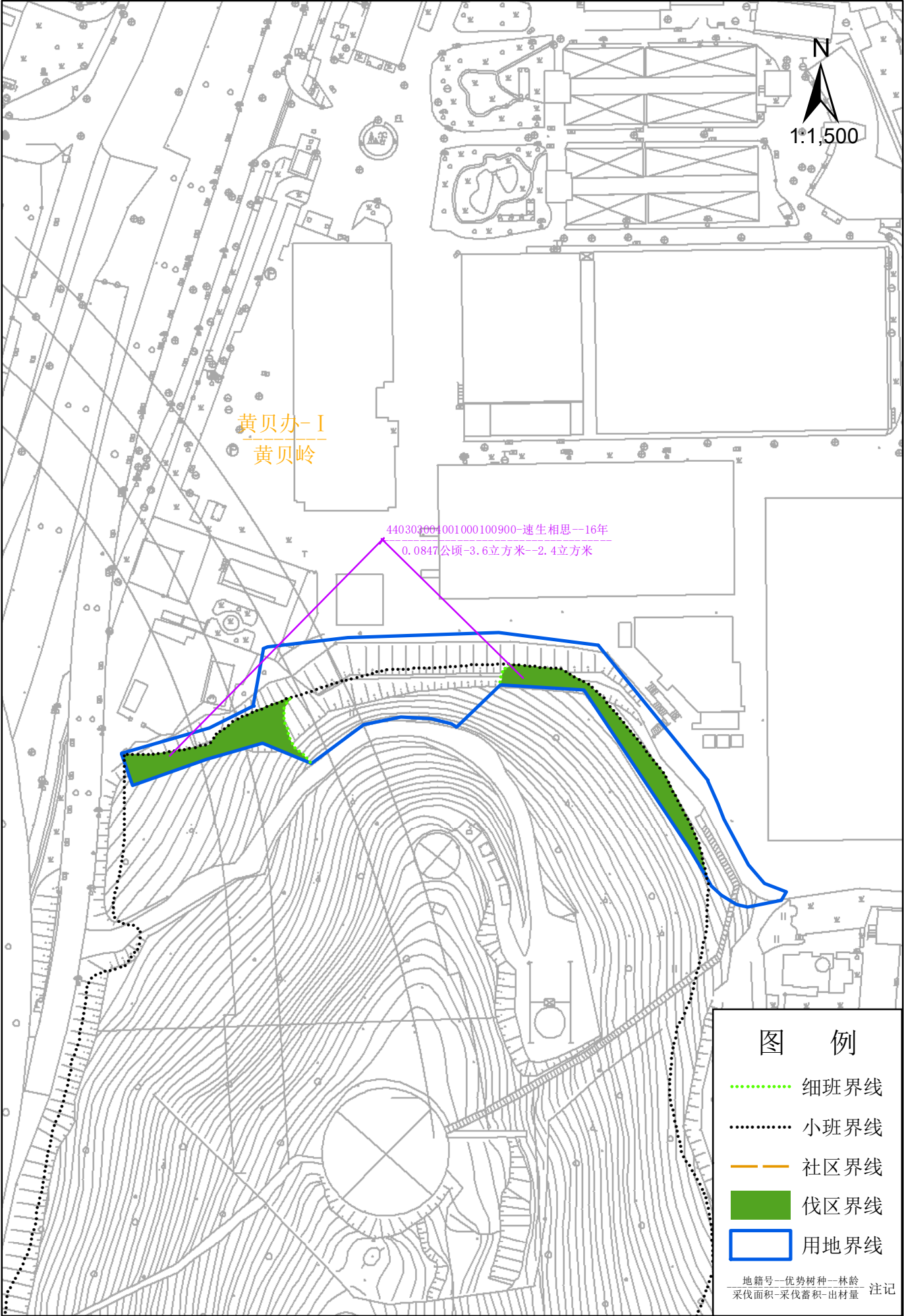
深圳东湖水厂扩能改造工程（南侧边坡治理工程）伐区位置基本图
