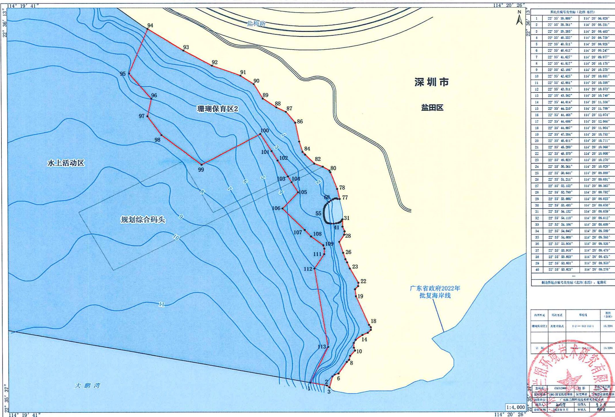
小梅沙海洋游憩公共设施(珊瑚保育区2)宗海界址图
