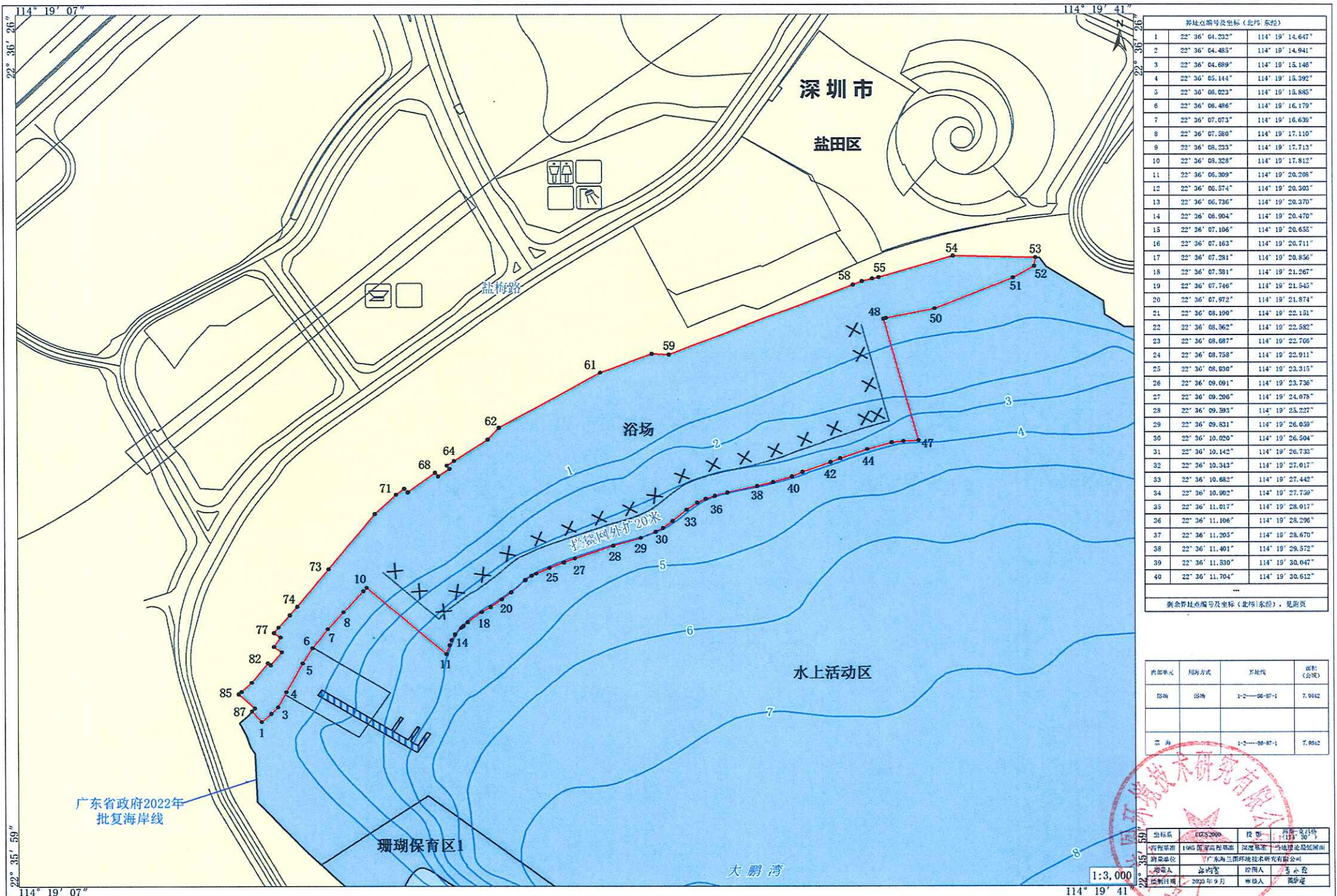
小梅沙海洋游憩公共设施(浴场)宗海界址图
