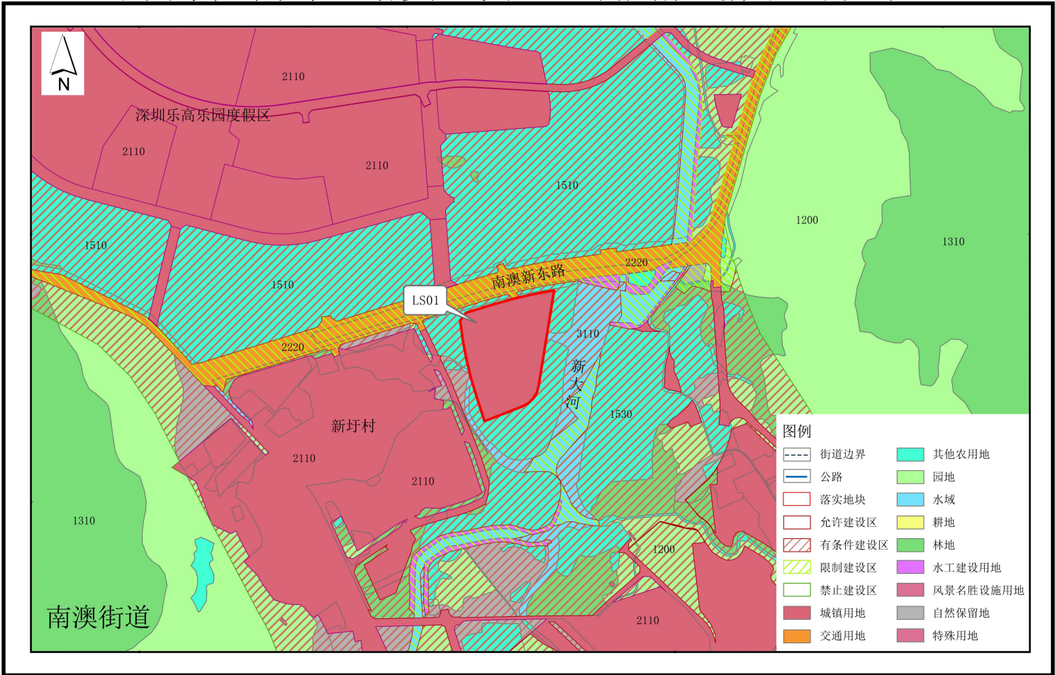
深圳市龙岗片区落实地块土地利用规划图（调整后）
