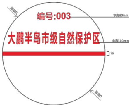
图 F.1 水域界桩设计图
