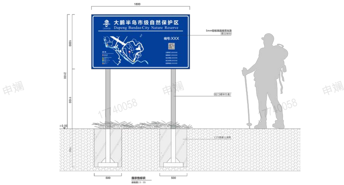
图 D.2 指示性标识牌设计图
