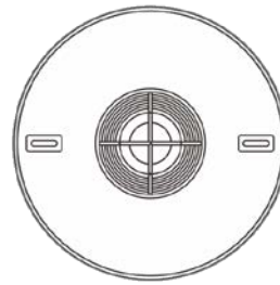
水域界桩（柱形） 俯视图 | 1:20
