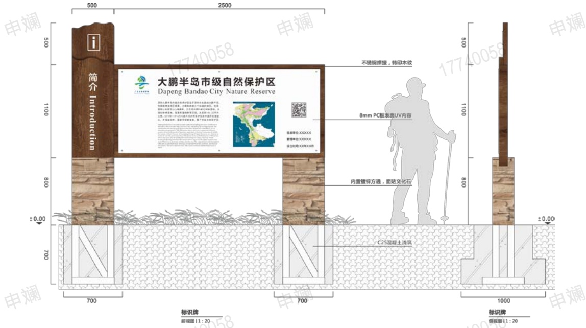
图 D.1 标识牌设计图
