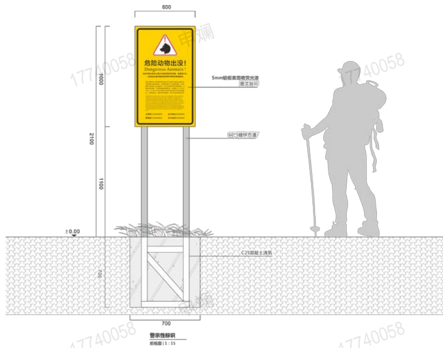
图 D.3 警示性标识牌设计图
