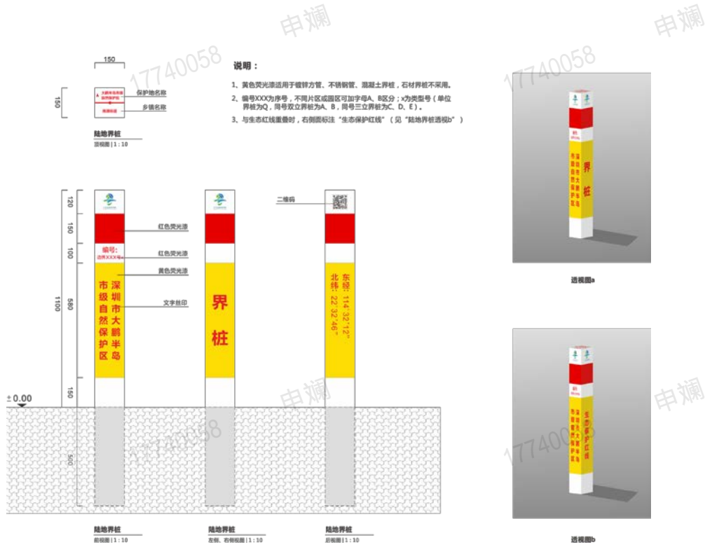
图 F.1 陆地界桩设计图
