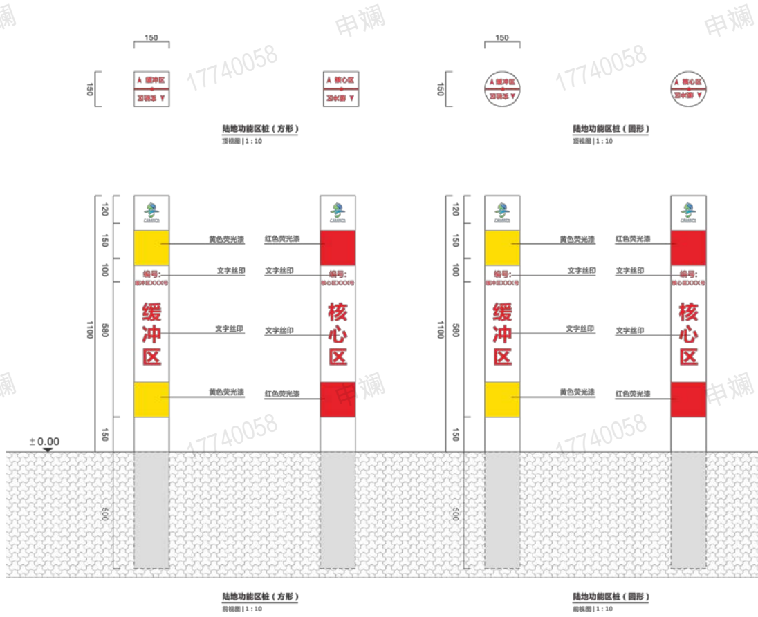
图 G.1 功能区桩设计图
