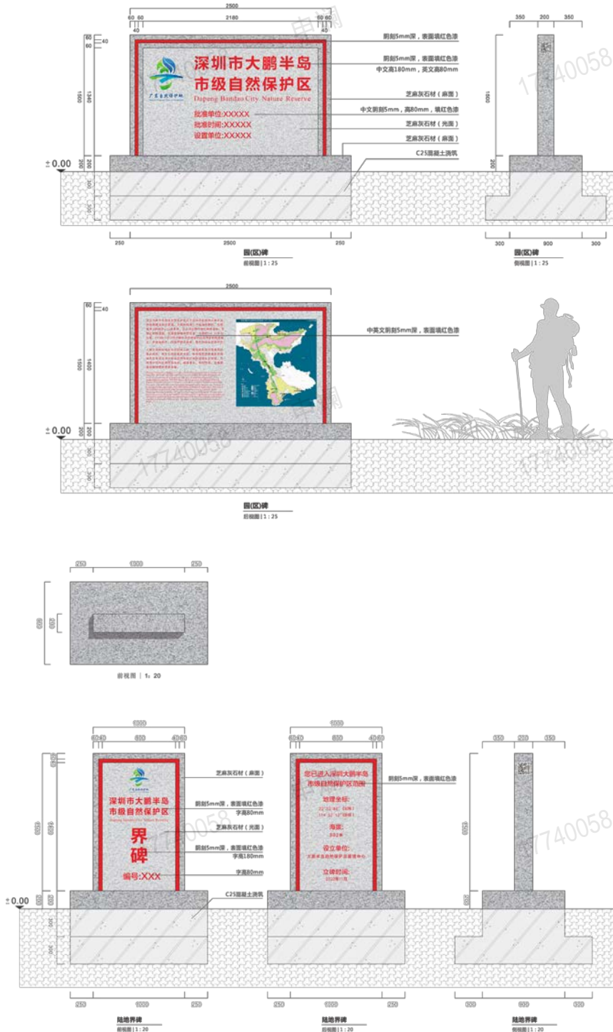
图 E.1 区(园)碑、界碑设计图
