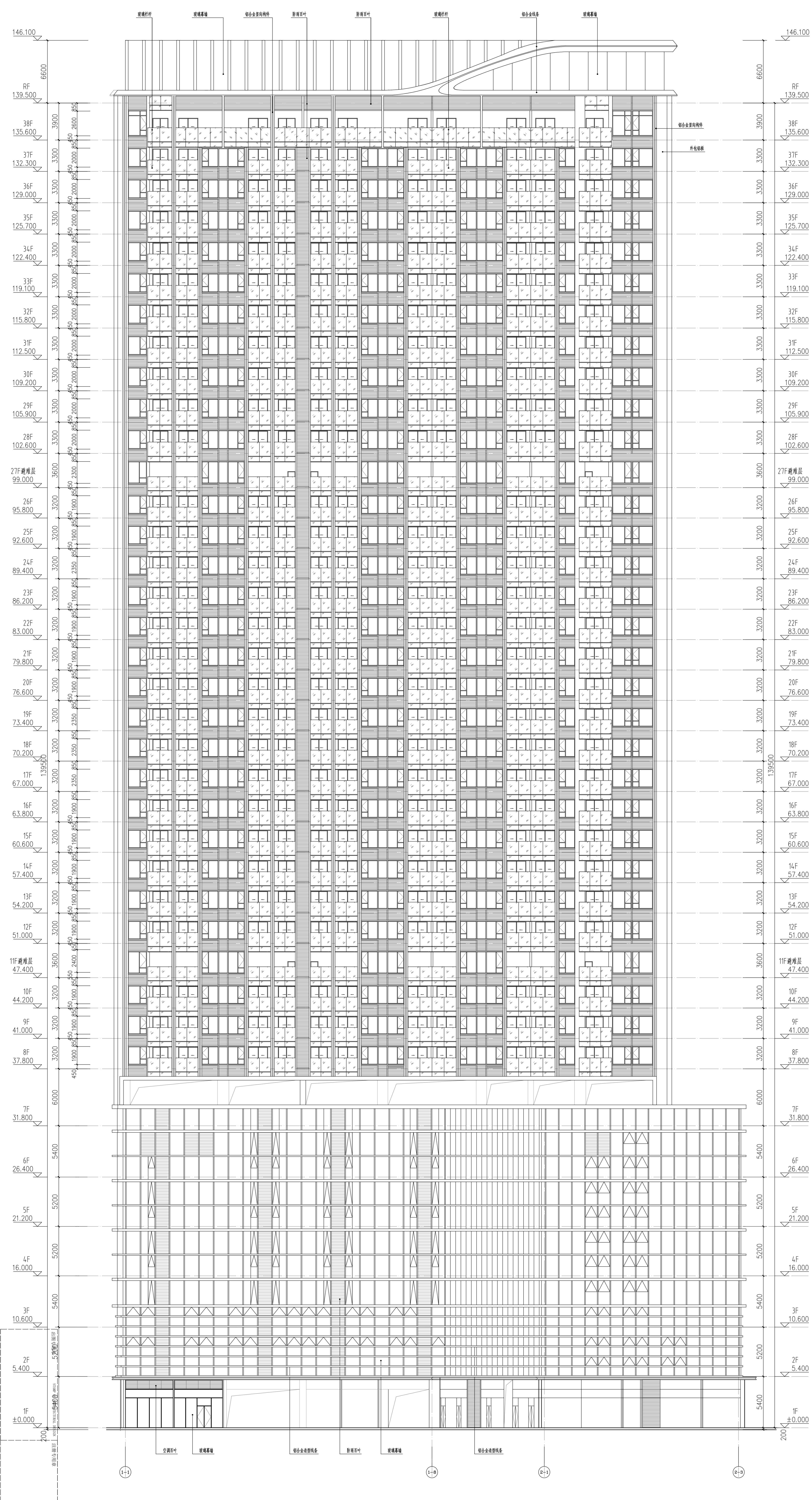
1-1 2-4 轴立面图 1:100
